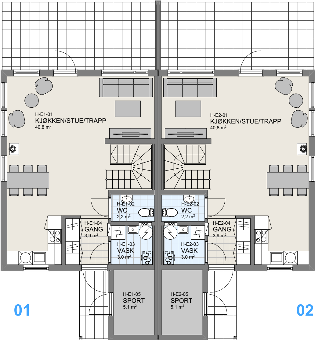
1:100 H. Etasje
