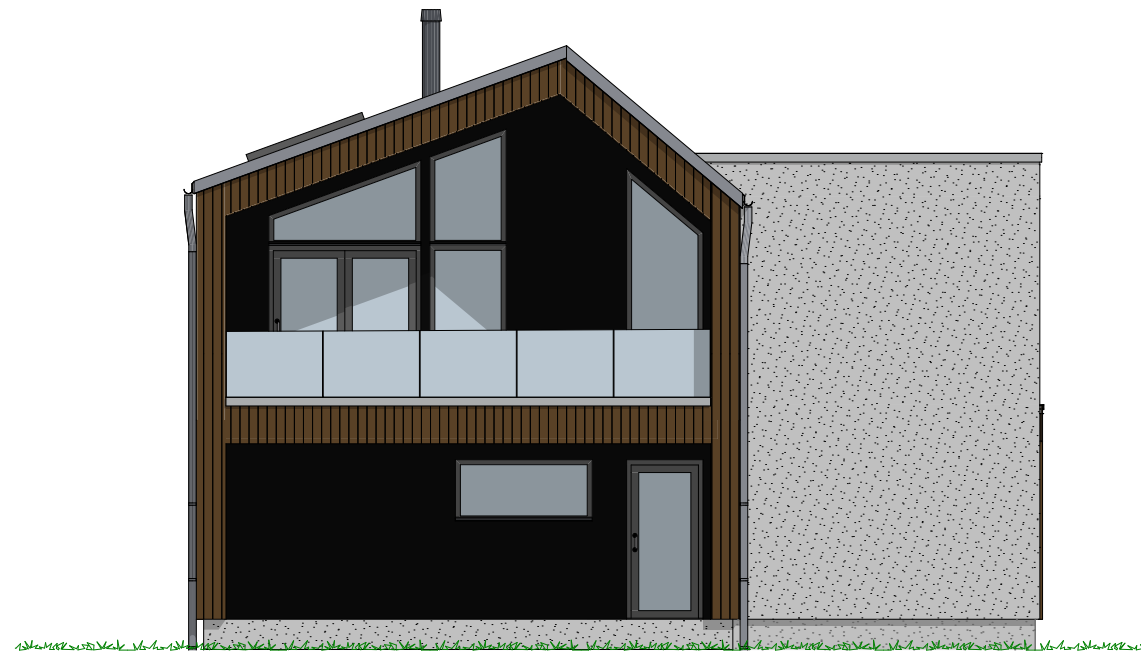
1:100 Fasade Nord
