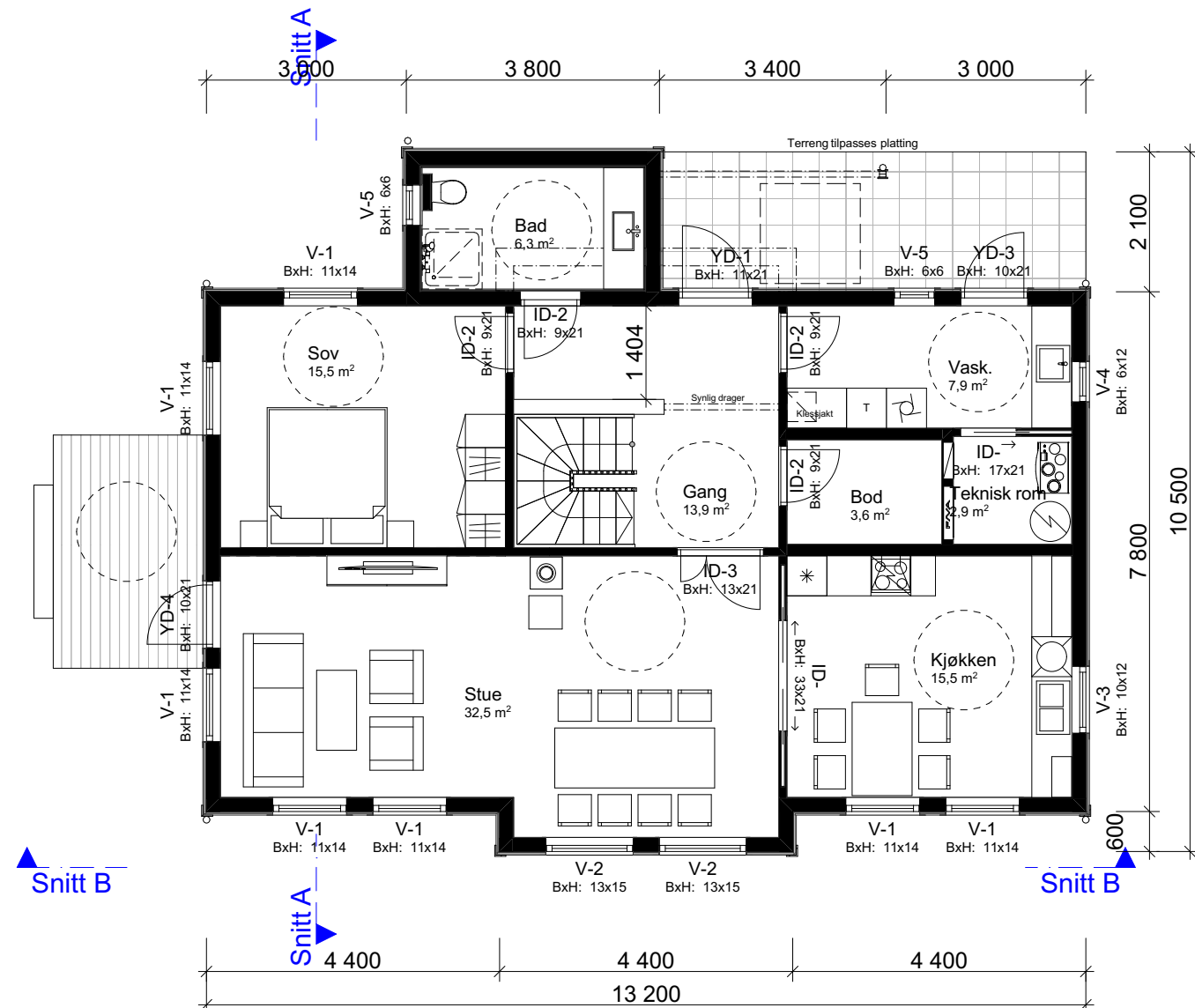
1:100 H. Etasje
