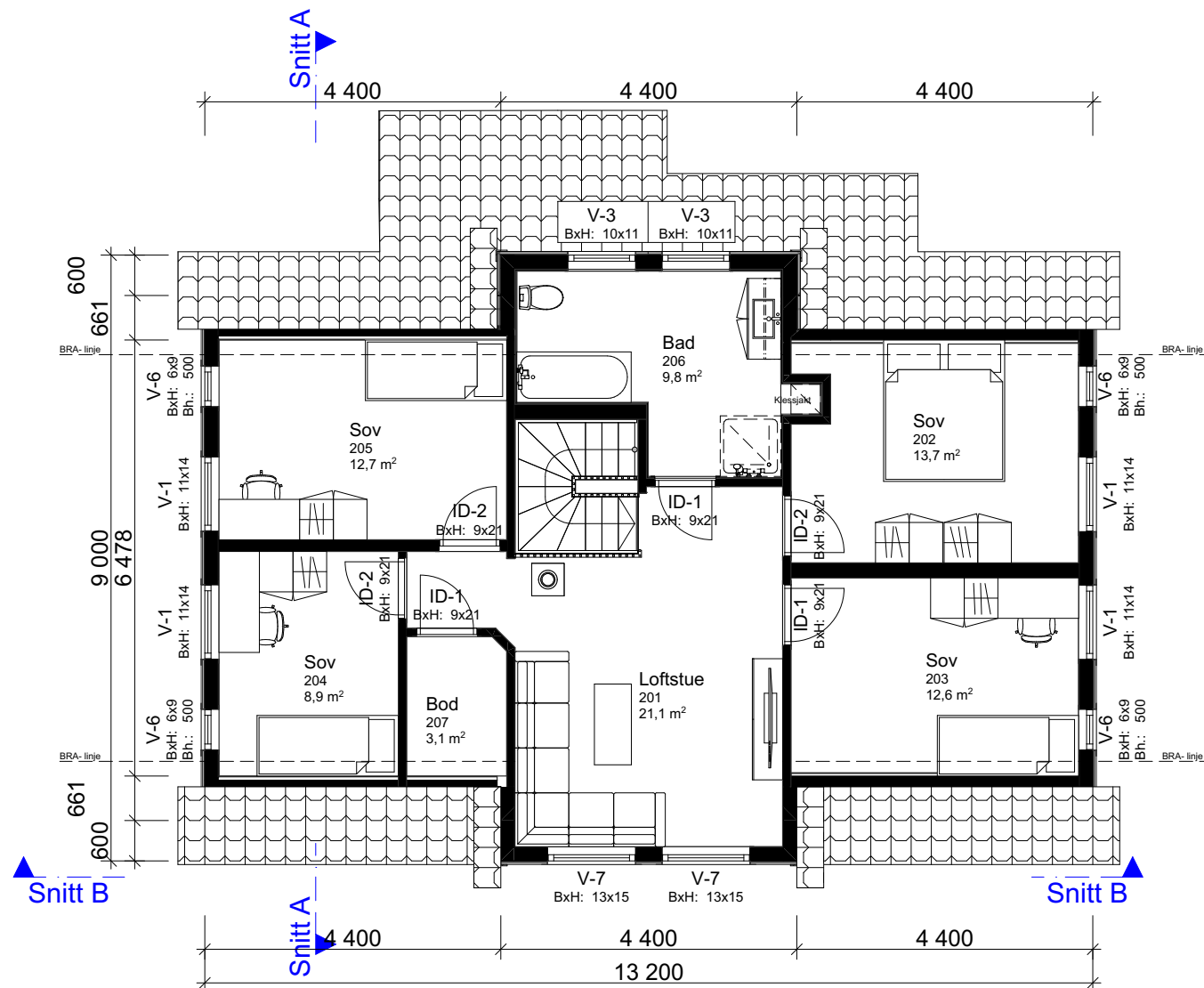
1:100 2.Etasje
