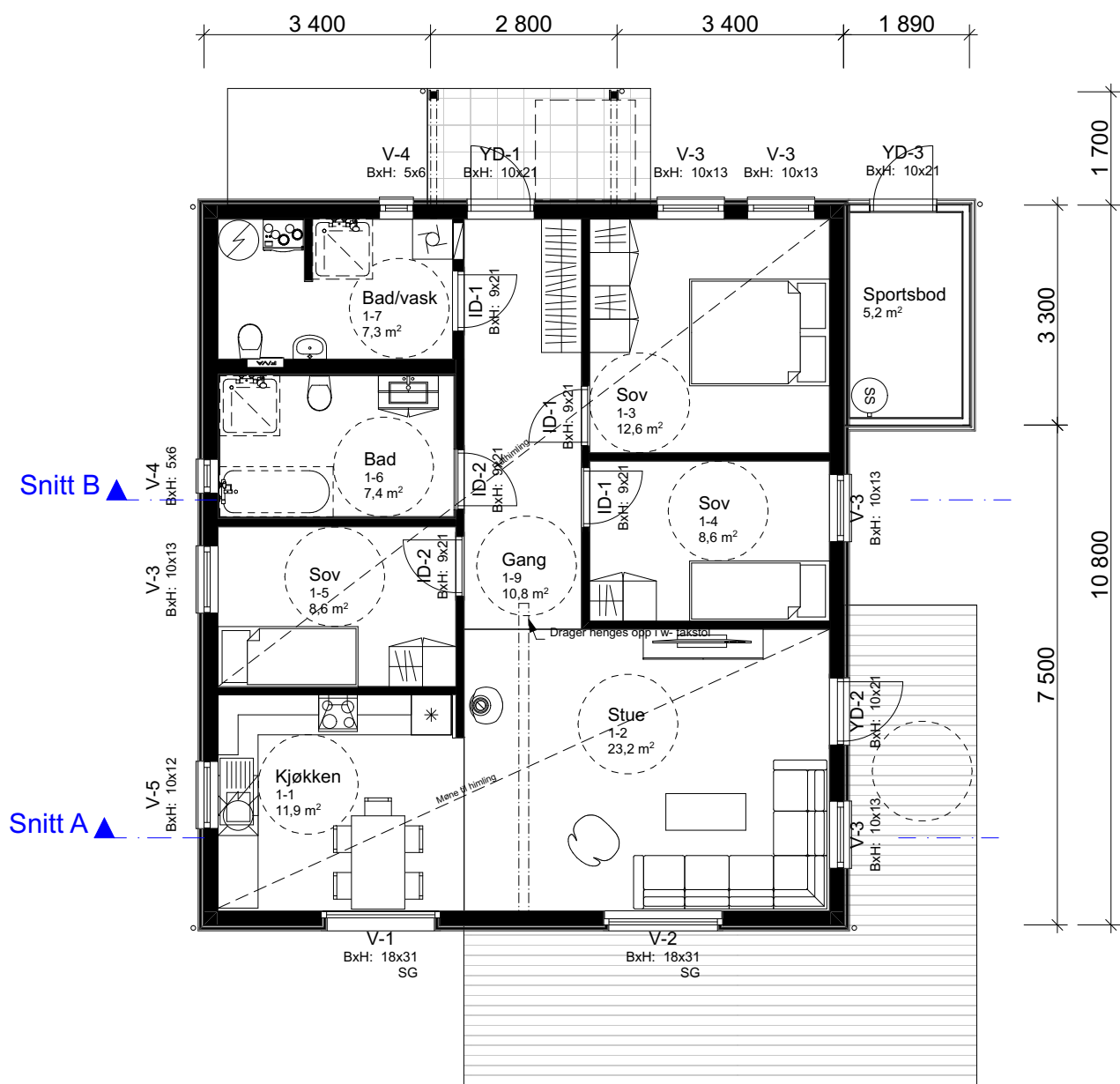
1:100 H. Etasje
