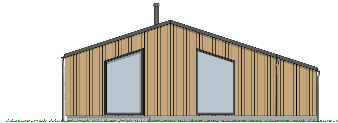
1:100 Fasade Vest
